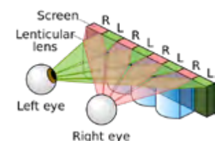
Funktions-Schema von Lentikularlinsensystemen: das linke Auge sieht immer einen anderen Blickpunkt wie das Rechte
