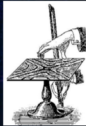
Formation d'une figure de Chladni par un archet.
